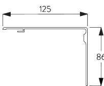
SG 8678 Cache de boîte encastré 105x125 mm
