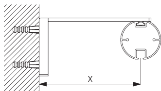
Smart Fix avec fente SG 11206 - SG 11208 et support SG 6141: Vis SG 20798 (M4x10) nécessaire.
